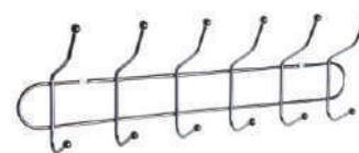
103178 Крючок на планке шестерной "C206", хром L75 x W515 x H165
